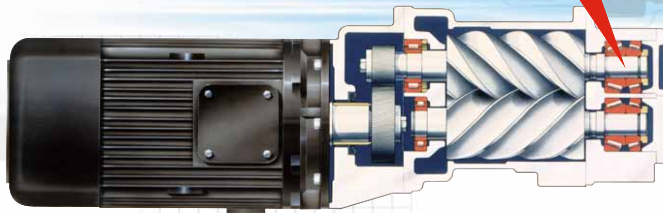
DIGA REFRIGERANTE CUSCINETTO
